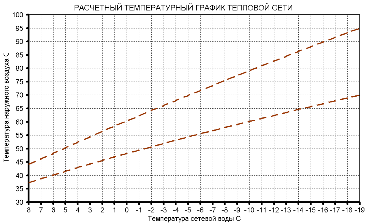
Рисунок 4. Расчетный температурный график тепловых сетей
